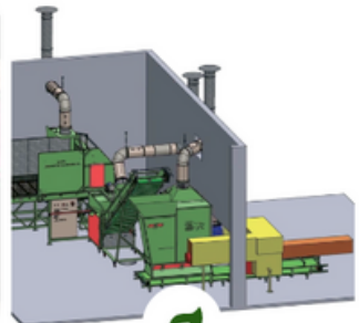
Anlage zum Heuumpressen
